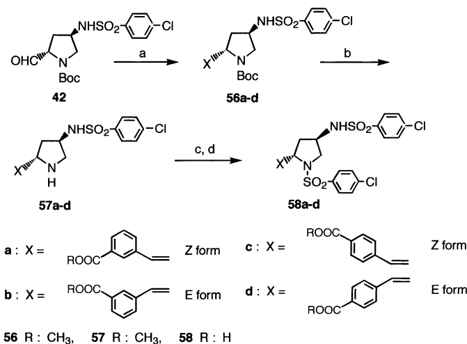
Scheme 6. (a) Ph 3 P + Cl - CH 2 Ph - ( m - or p -)COOMe, NaH, THF; (b) 90% TFA; (c) p -Cl-PhSO 2 Cl, Et 3 N, CH 2 Cl 2 ; (d) 1N-NaOH, MeOH.
