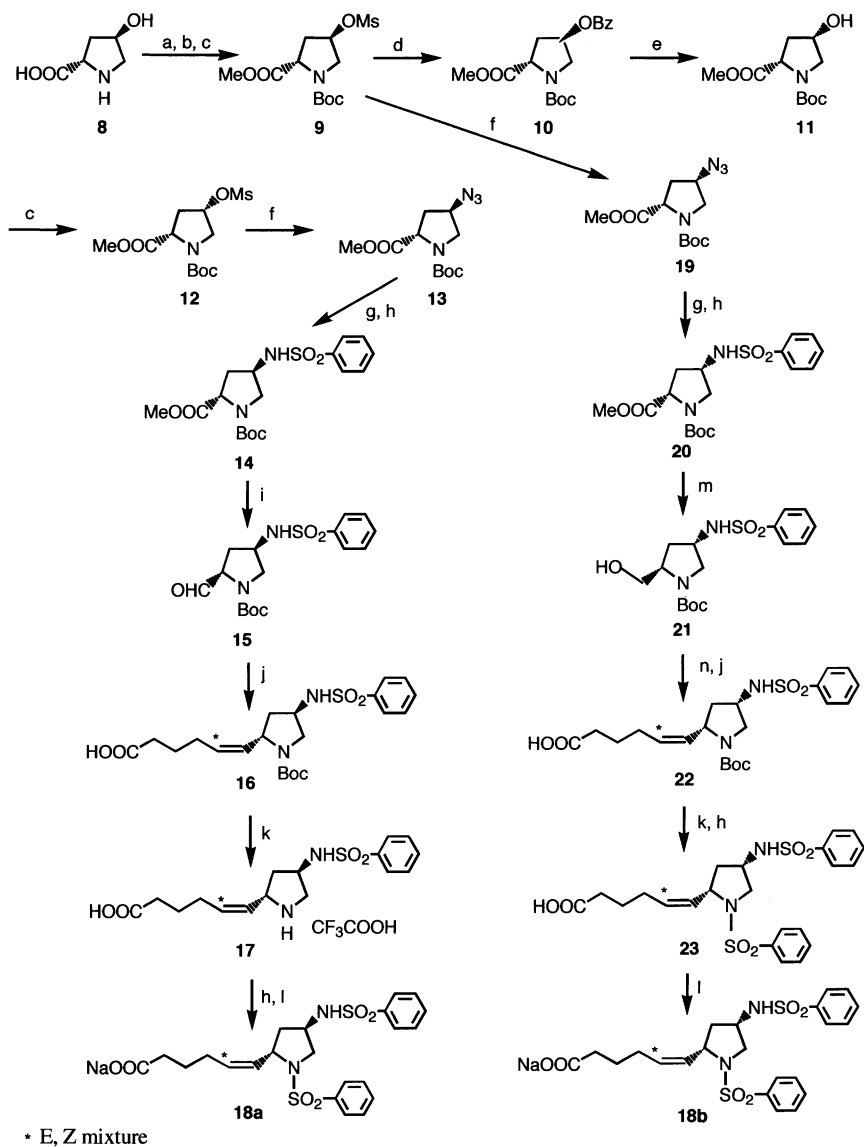
Scheme 2. (a) SOCl 2 , MeOH; (b) Boc 2 O, Et 3 N, CH 2 Cl 2 ; (c) MsCl, Et 3 N, CH 2 Cl 2 ; (d) BzONa, DMSO; (e) K 2 CO 3 , MeOH; (f) NaN 3 , DMSO; (g) H 2 -Pd/C, MeOH; (h) PhSO 2 Cl, Et 3 N, CH 2 Cl 2 ; (i) DIBAL, toluene, -78 °C; (j) HOOC(CH 2 ) 4 P + Ph 3 Br - , t -BuOK, DMAC; (k) 75% TFA; (l) 1N-NaOH, MeOH; (m) DIBAL, toluene, -25 °C; (n) CrO 3 , pyridine, CH 2 Cl 2 .
