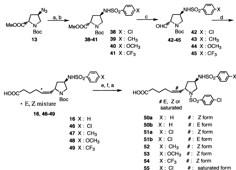
Scheme 5. (a) H 2 -Pd/C, MeOH; (b) p -XPhSO 2 Cl, Et 3 N, CH 2 Cl 2 ; (c) DIBAL, CH 2 Cl 2 ; (d) HOOC(CH 2 ) 4 P + Ph 3 Br - , t -BuOK, DMAC; (e) 75% TFA; (f) p -ClPhSO 2 Cl, Et 3 N, CH 2 Cl 2 .
